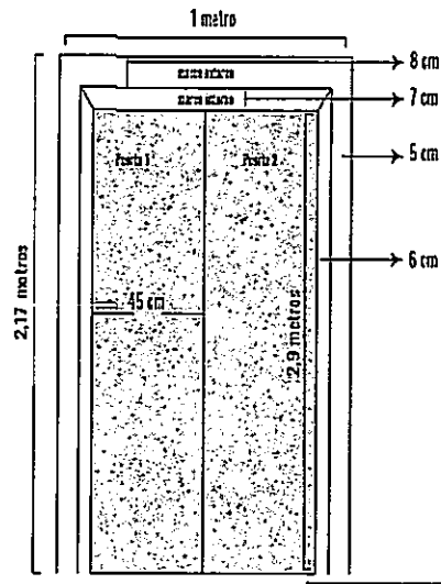
MARCOS - PUERTAS ASCENSOR DEL SOTANO AL PISO 8
