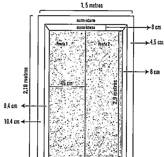
MARCOS - PUERTAS ASCENSOR PISO 9
